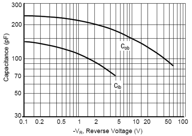
Fig. 4 Capacitance
