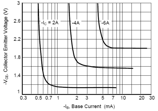
Fig. 2 V_{CE} vs. I_B
